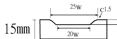
溝拡大図
